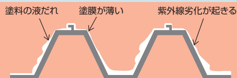
折板屋根断面図
